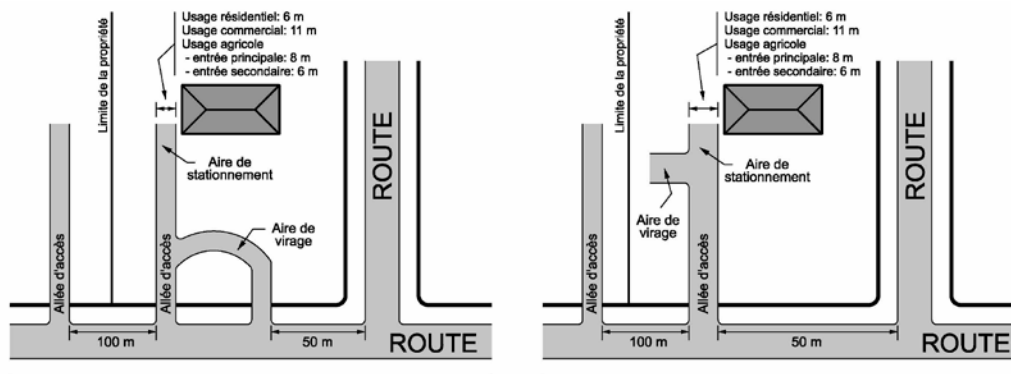
Croquis 11.4 Aménagement des aires de stationnement et allées d'accès en bordure d'une route du réseau supérieur à l'extérieur du périmètre d'urbanisation
