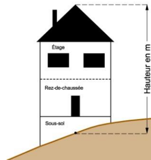
Croquis 6.4 Hauteur d'un bâtiment en mètre
