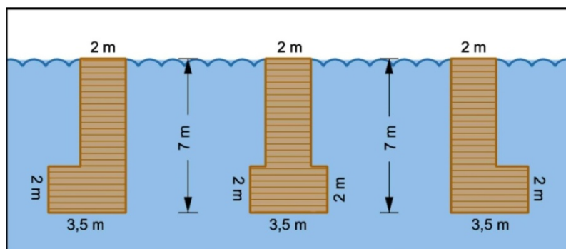
Croquis 13.3 Formes et dimensions des quais
