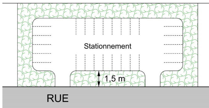
Croquis 11.2 Aménagement des espaces verts à l'intérieur d'une aire de stationnement
