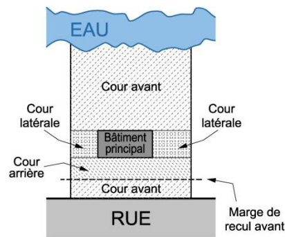
Croquis 2.5 Localisation des cours pour un bâtiment situé sur un terrain adjacent à un lac ou à un cours d'eau
