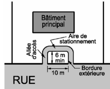
Croquis 11.3 Aménagement d'une aire de stationnement en « U » devant la façade d'un bâtiment principal
